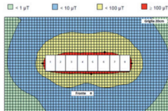
Figura 5.6: Rappresentazione grafica del campo magnetico (caso peggiore) intorno al QMT, visto dall'alto
