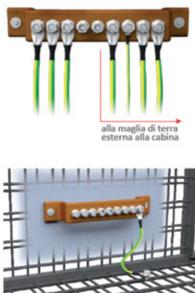
Figura 1.17: Collegamento impianto di terra
